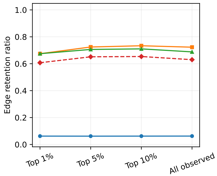
M=16
