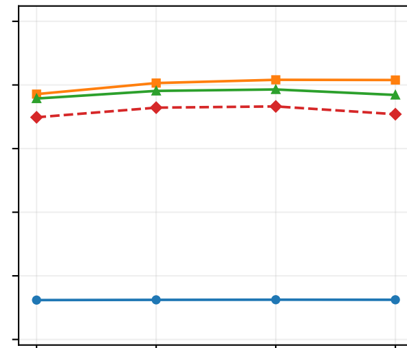
M=8
