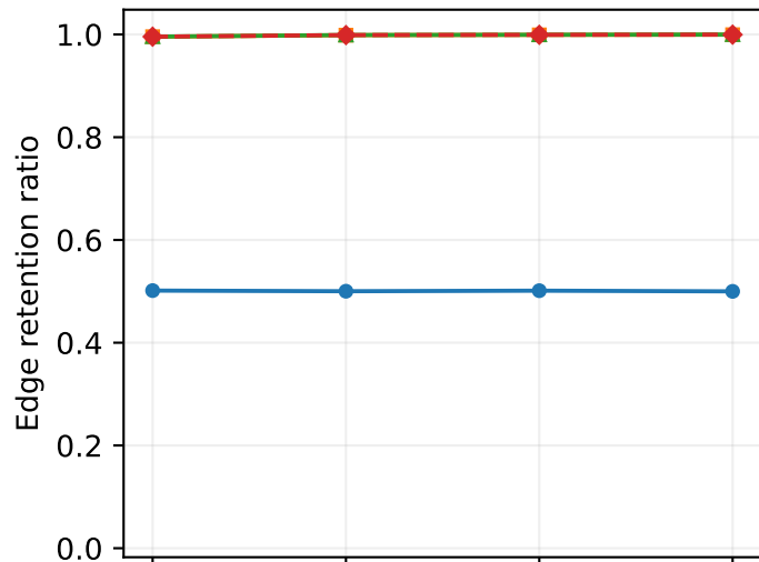
M=16
