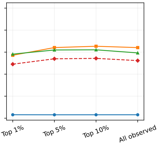
M=32
