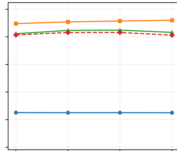
M=32
