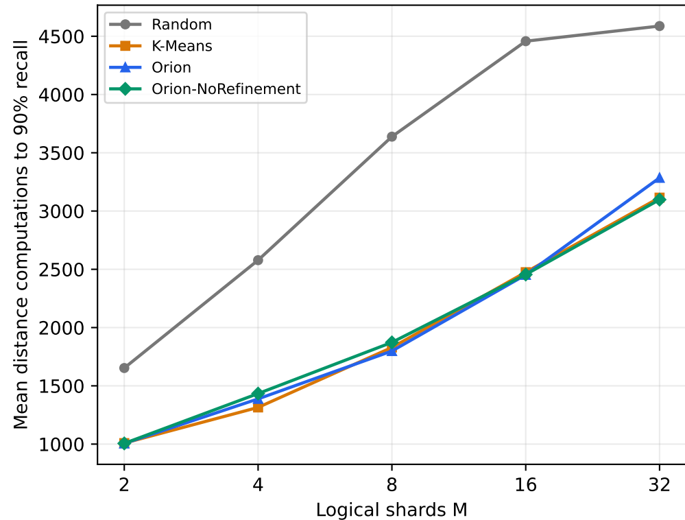
SIFT1M
