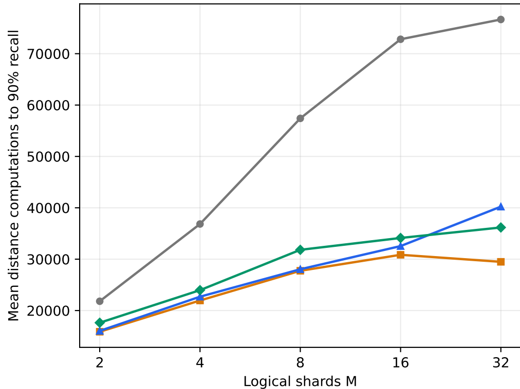
GloVe-200
