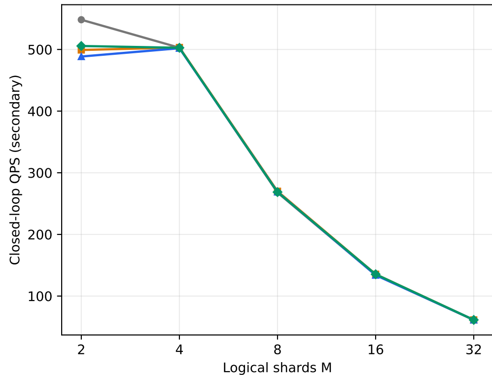
GloVe-200
