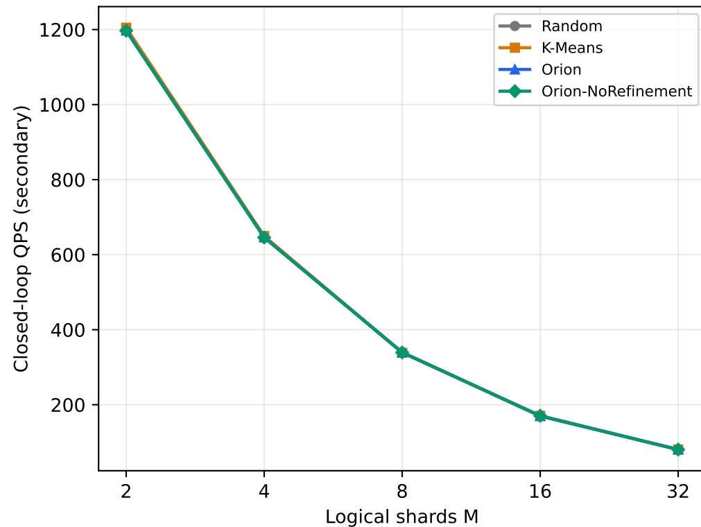
SIFT1M
