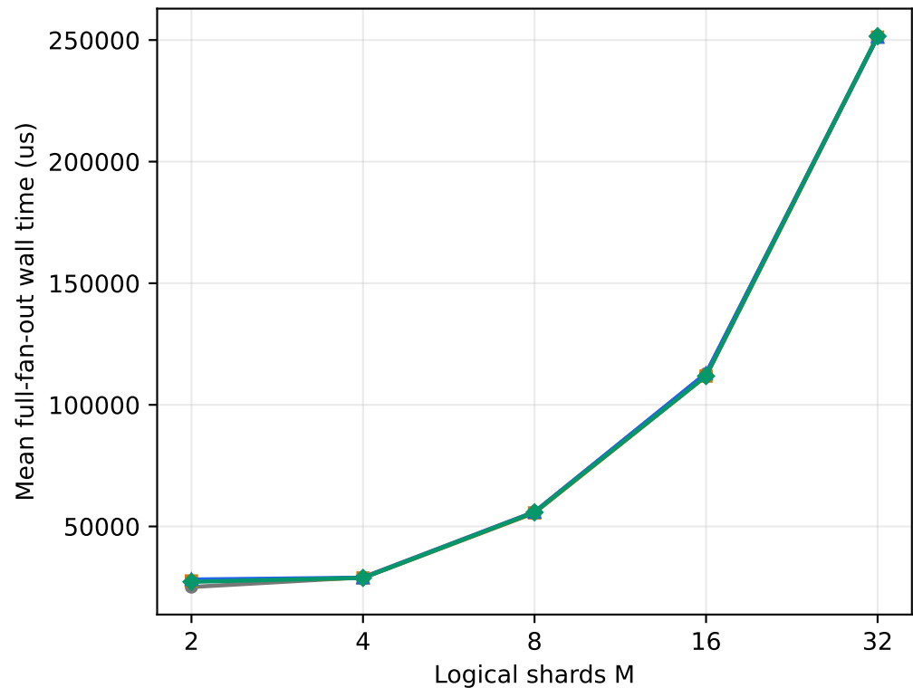
GloVe-200
