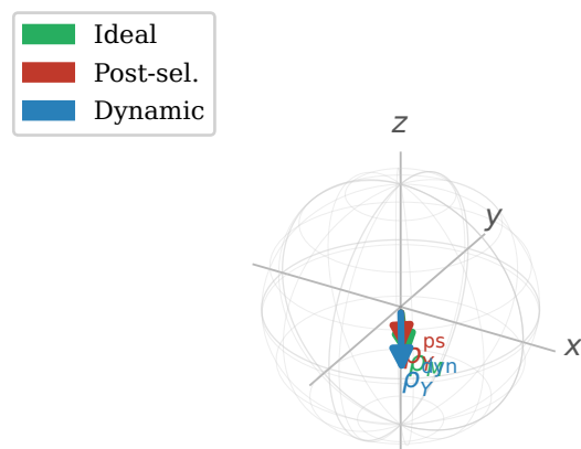
(d) Bloch sphere
