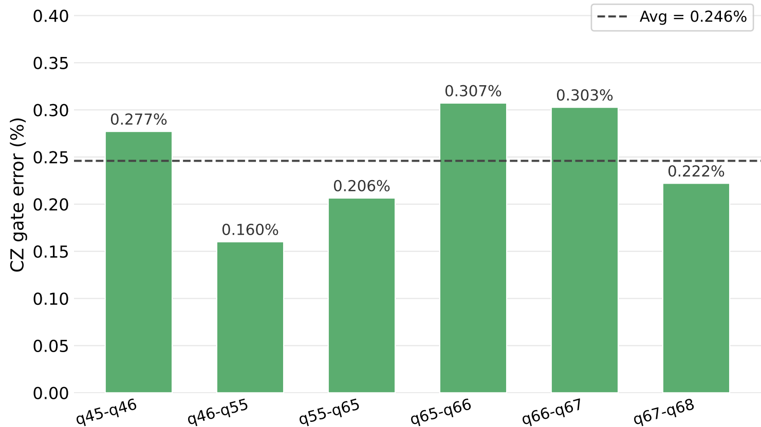
(b) ibm_torino - CZ gate error rates per edge
