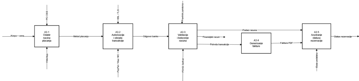
Slika 9 – IDEF0 A3: Detaljna dekompozicija obrade plaćanja
