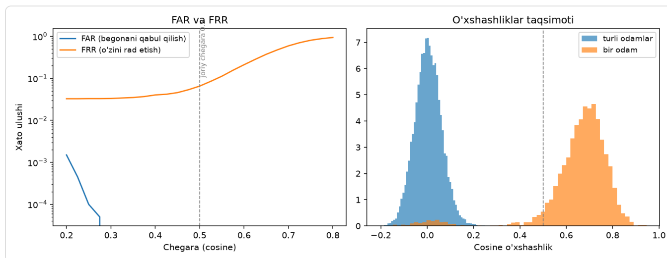
FAR va FRR egri chiziqlari hamda o'xshashliklar taqsimoti (LFW)
