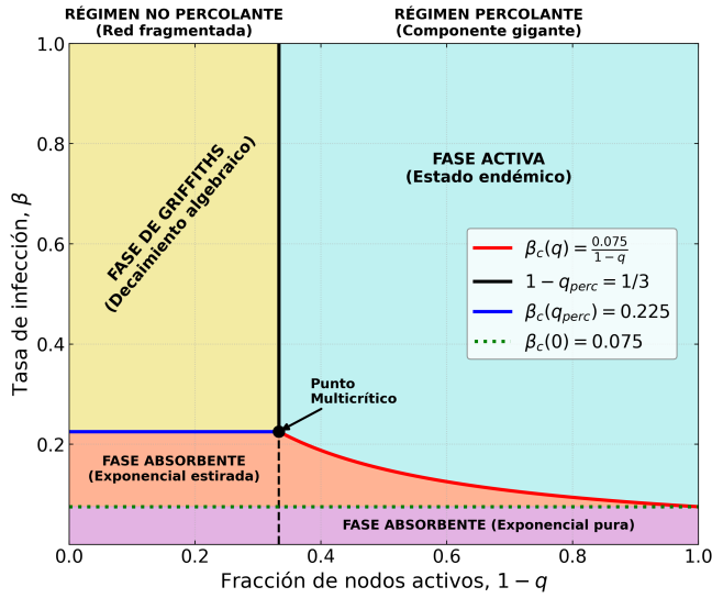
Figura 7. Diagrama de fases teórico DBMF para el modelo SIS con desorden bimodal ( \langle k \rangle = 3 , \mu = 0.3 ). La línea negra continua marca el umbral de percolación q_{perc} = 2/3 , dividiendo el sistema en un régimen de componente gigante y un régimen fragmentado.
