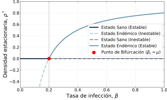
Figura 1. Diagrama de bifurcación transcítica en la aproximación de campo medio del modelo SIS. En \beta_c = \mu / \langle k \rangle , la rama de \rho^* = 0 pierde estabilidad en favor del estado endémico. Para esta representación ilustrativa, se ha asumido un grado medio normalizado \langle k \rangle = 1 y una tasa de recuperación \mu = 0.2 , situando el punto de bifurcación en \beta_c = 0.2 .
