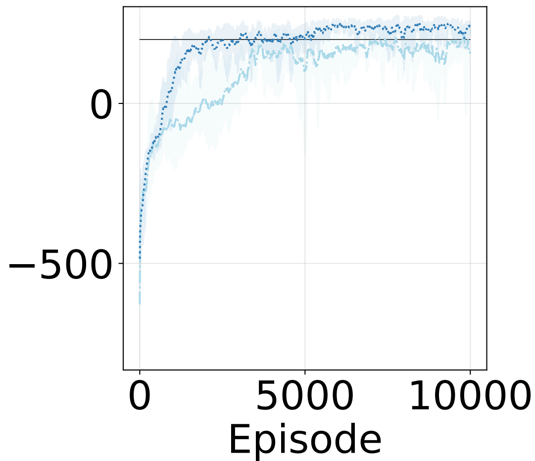
LunarLander-v3
