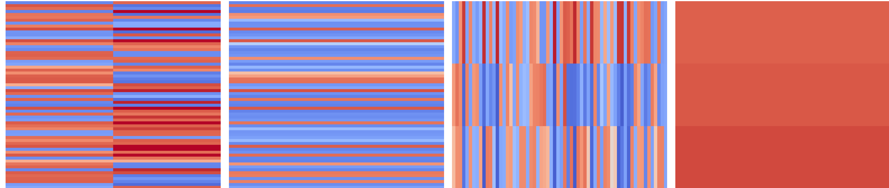
W_1 (2 X 64)
