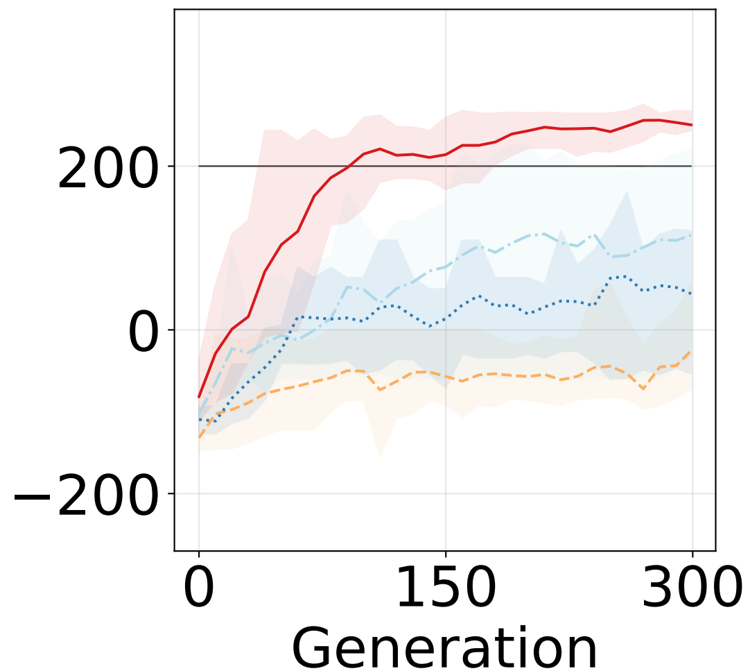
LunarLander-v3
