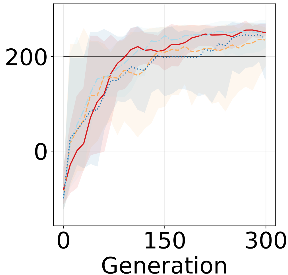
LunarLander-v3
