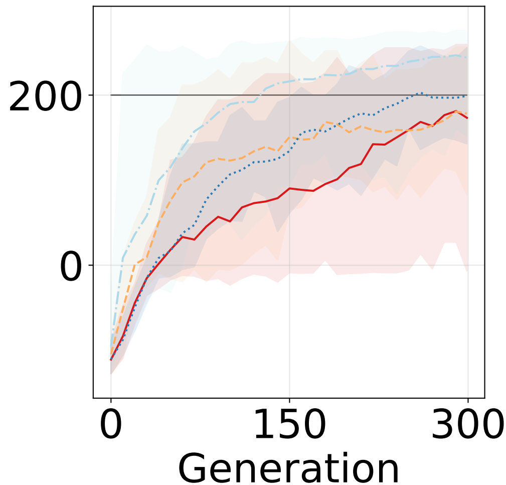
LunarLander-v3
