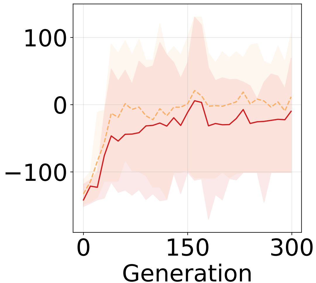
LunarLander-v3
