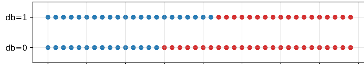
N=10 | Siegert FP enumeration | J(db=0)=0.00, J(db=1)=0.00
