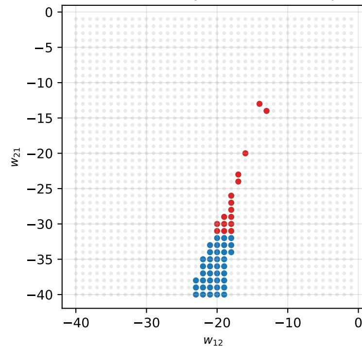
N=20000: 54 Siegert-blue → QR-red flips
