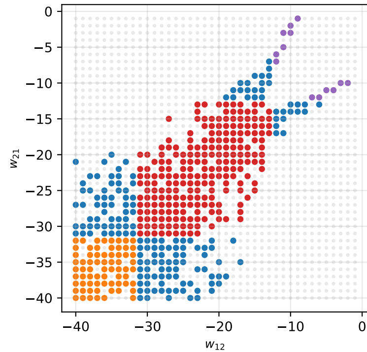
N=2000: 55 Siegert-blue → QR-red flips
