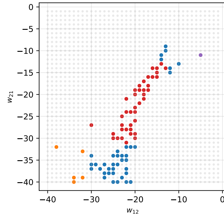
N=100: 84 Siegert-blue → QR-red flips
