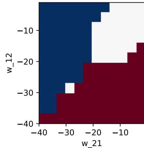
LI&amp;F oracle
