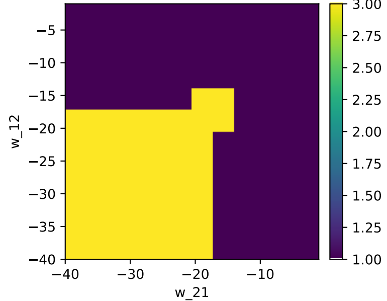
Siegert # fixed points
