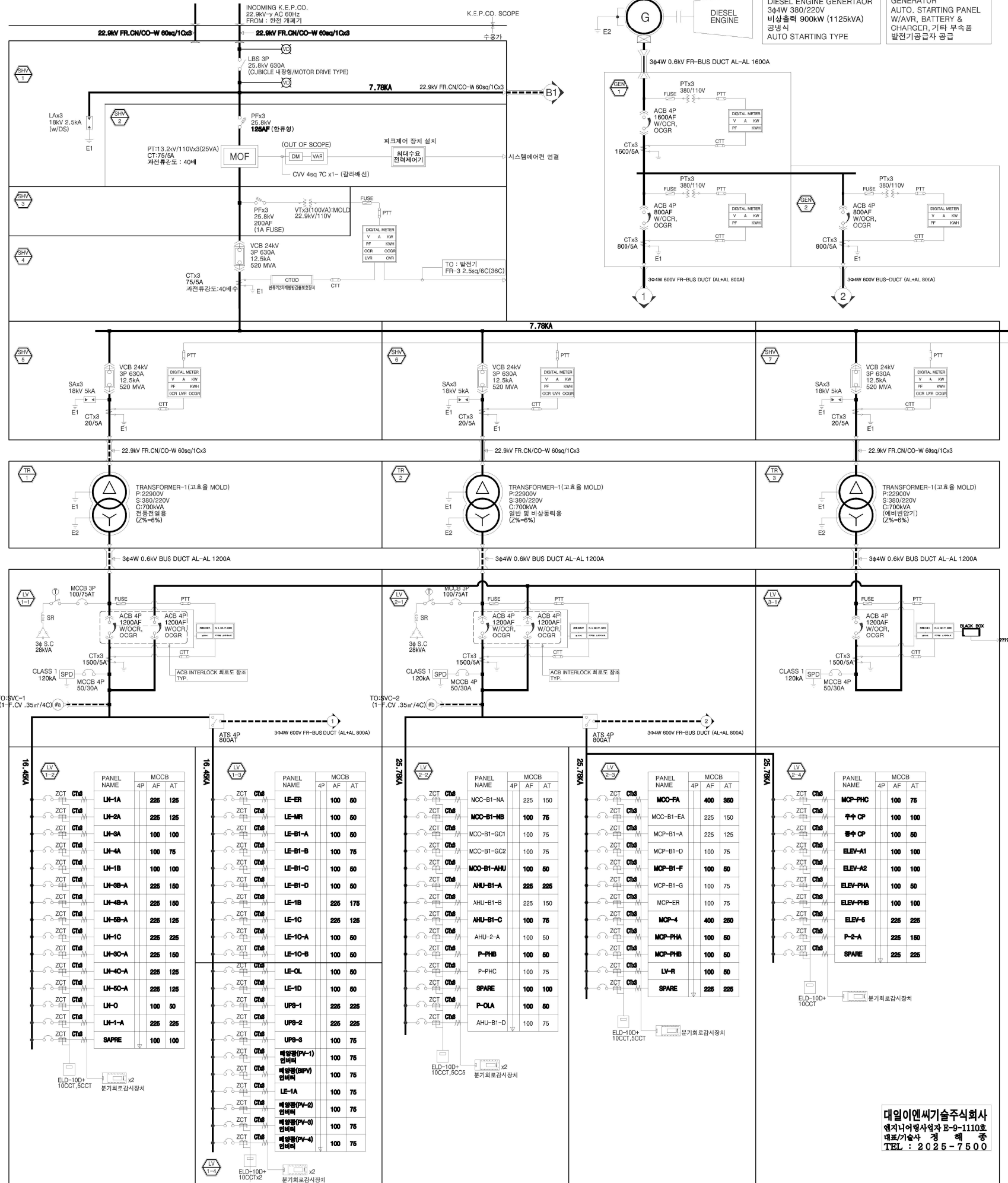
수변전설비 단선 결선도-1
