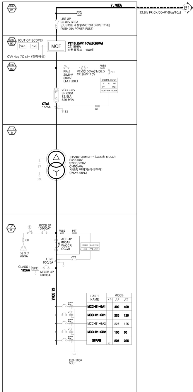
수변전설비 단선 결선도-1
