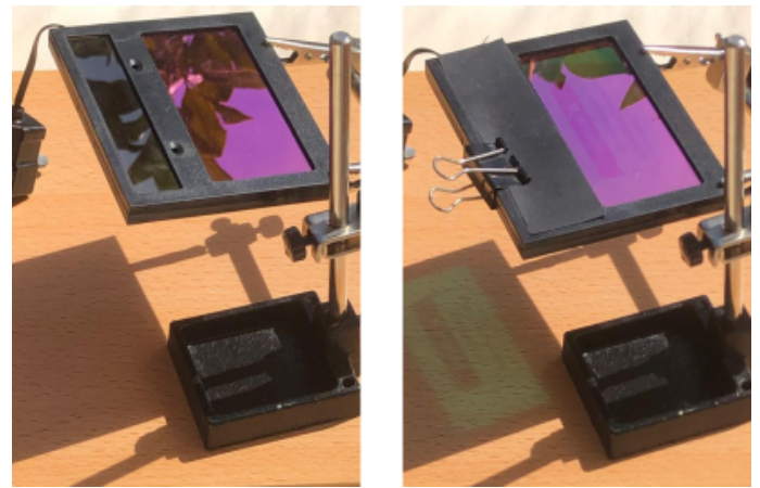
Figura 7: Quan el sensor de les ulleres de soldador queda exposat directament al Sol, el filtre de cristall líquid s'enfosqueix i bloqueja bona part de la llum. Si tapem el sensor amb una cartolina, el filtre deixa d'activar-se i torna a deixar passar la llum; això es pot veure a la zona verda de la part inferior. Imatge creada per l'autor, CC BY 4.0.
