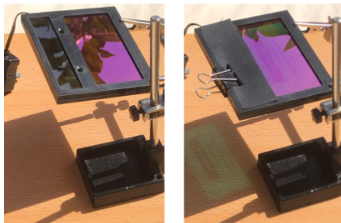
Figura 7: Quan el sensor de les ulleres de soldador queda exposat directament al Sol, el filtre de cristall líquid s'enfosqueix i bloqueja bona part de la llum. Si tapem el sensor amb una cartolina, el filtre deixa d'activar-se i torna a deixar passar la llum; això es pot veure a la zona verda de la part inferior. Imatge creada per l'autor, CC BY 4.0.
