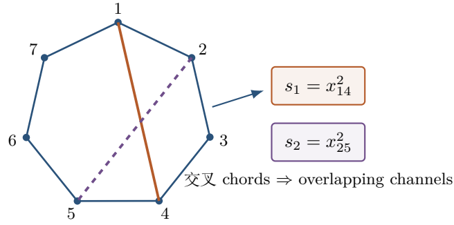
图 13.1: 七边形中相交 chords 表示一对 overlapping three-particle channels。相应 first-entry double discontinuity 受 Steinmann relation 禁止。
