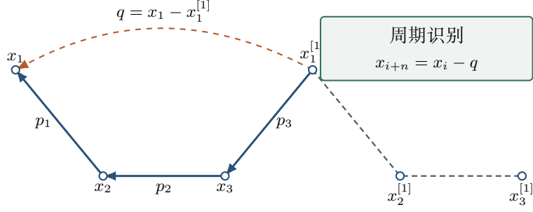
图 6.1: form factor 的周期 dual polygon。实线是一个基本域，灰色虚线是下一周期像；橙色虚箭头表示局域算符注入的 off-shell 动量 q 。
