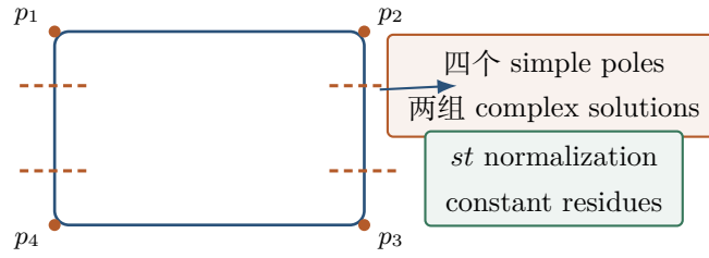
图 12.2: normalized box 的 quadruple cut 与 d\log 性质。橙色角点表示 tree amplitudes, 虚线表示 cut propagators。
