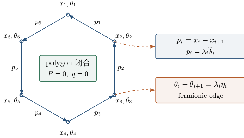
图 3.1: planar 六点 dual superpolygon。外部 on-shell 数据成为相邻区域点之间的边；周期条件把总动量与总超动量守恒几何化。
