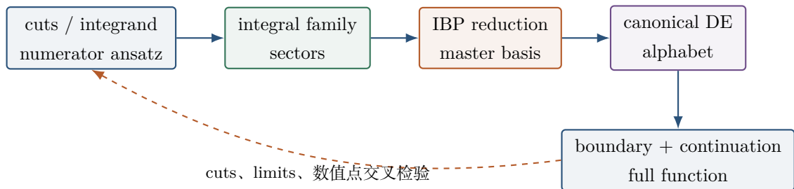
图 12.1: 从 rational integrand 到完整多圈函数的四层流水线。每个箭头都需要独立的 basis、boundary 或 regulator 选择。
