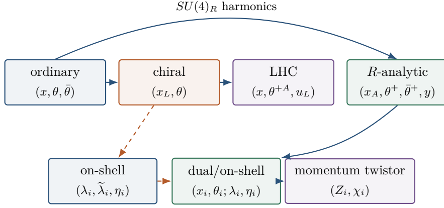
图 3.2: ordinary、analytic、LHC、on-shell、dual 与 momentum-twistor superspace 的操作字典。箭头表示有条件的构造或映射，而非无条件同构。
