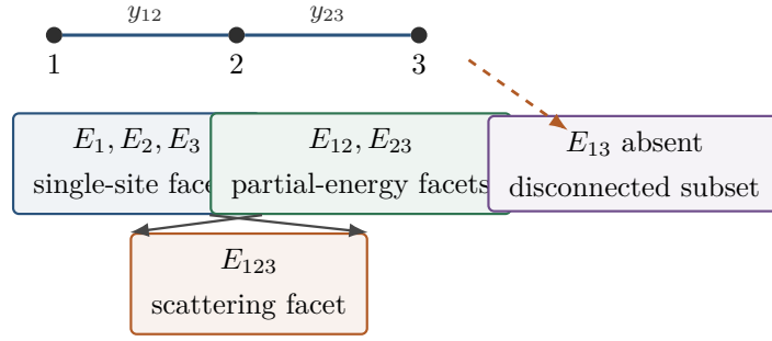
图 14.1: 三 site chain 的能量 pole atlas。图的连通性决定允许的 primitive facets; 不存在 E_{13} 是一条非平凡解析约束。
