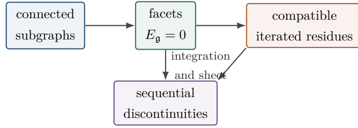
图 14.2: 从 graph combinatorics 到积分后 discontinuities 的层级。竖直箭头依赖积分与 branch prescription，不能仅由 face lattice 自动完成。
