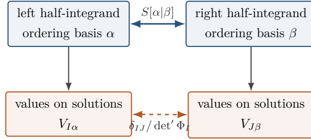
图 10.3: KLT orthogonality 的线性代数字典。ordering basis 与 solution basis 由 PT evaluation matrix 联系。
