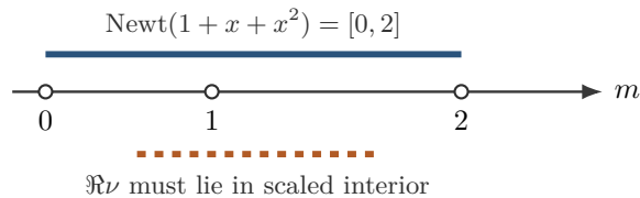
图 9.3: 一变量 Newton polytope。端点对应积分的不同 asymptotic regions; 高维时端点推广为 facets。
