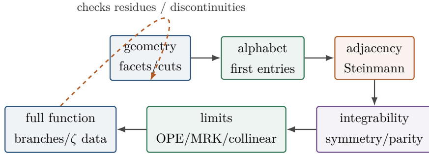
图 18.1: Geometry-informed bootstrap 的闭环。最后一步必须回查几何/物理 cuts，而不是只做 symbol 线性代数。
