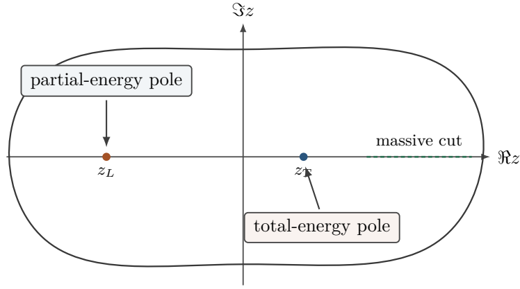
图 19.1: 一参数复形变后的奇点图。pole/cut 的位置取决于 c_a ；物理内容是它们对应的 total energy、partial energy 或 massive threshold，而不是图上的左右次序。
