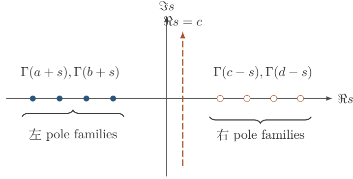
图 17.1: Mellin-Barnes contour 必须分开左右 pole families。参数解析延拓使两族 poles pinch 时, 不能仍沿原竖线积分而不补 residues。
