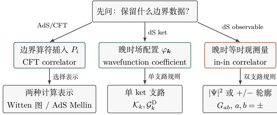
图 1: 对象选择树。方框区分“物理对象”与“计算表示”：Witten 图和 AdS Mellin amplitude 是 CFT 相关函数的两种组织；Schwinger–Keldysh 是 in-in 的双支路表示；dS 波函数系数则是缝合前的数据。由 \int \mathcal{D}\varphi \Psi \Psi^* 得到 in-in 观测量是另一步缝合，不在树图中画成交叉箭头。
