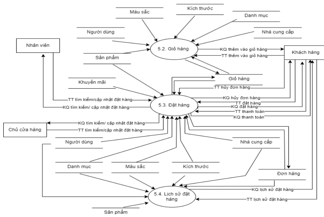
Hình 3.15. Sơ đồ luồng dữ liệu mức dưới đỉnh quản lý bán hàng
