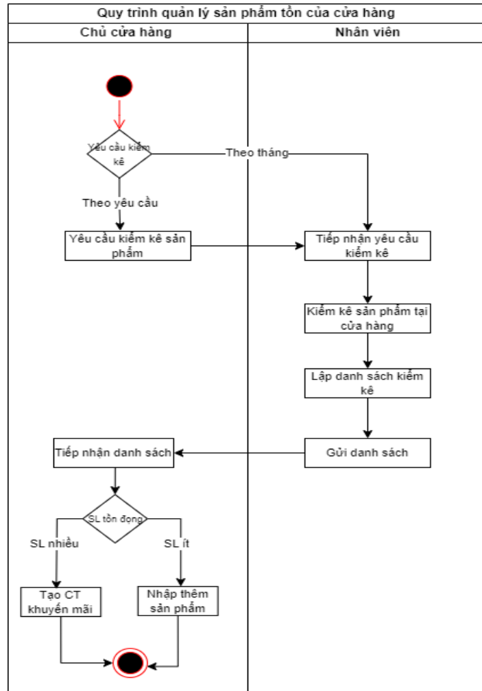
Hình 2.1. Quy trình quản lý sản phẩm tồn kho tại cửa hàng
