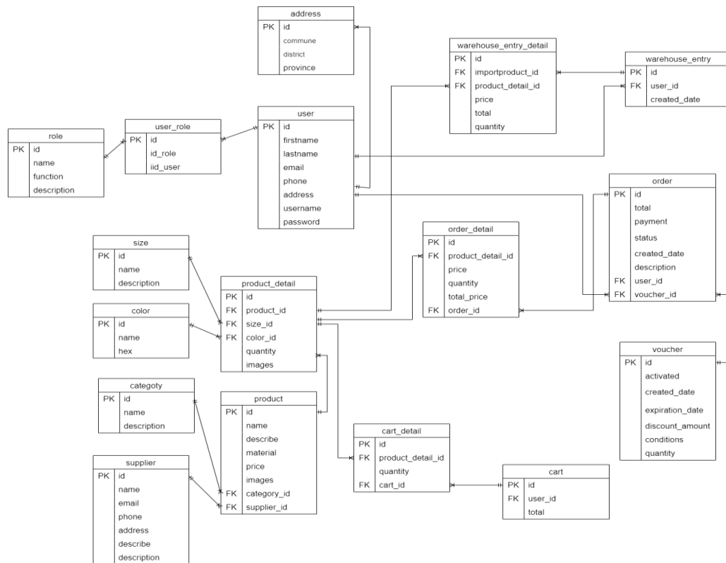
Hình 4.4. Sơ đồ quan hệ
