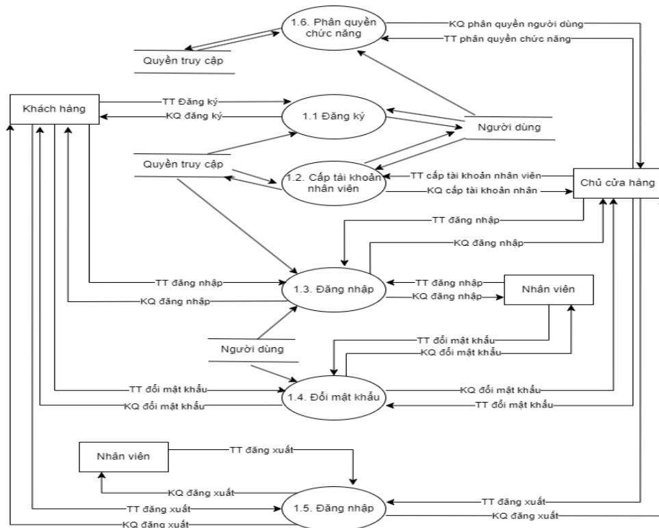
Hình 3.11. Sơ đồ luồng dữ liệu mức dưới đỉnh quản lý tài khoản
