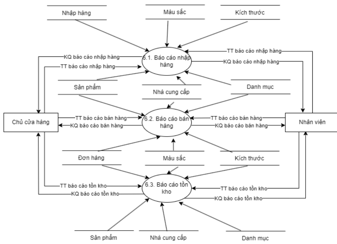
Hình 3.16. Sơ đồ luồng dữ liệu mức dưới đỉnh quản lý báo cáo thống kê
