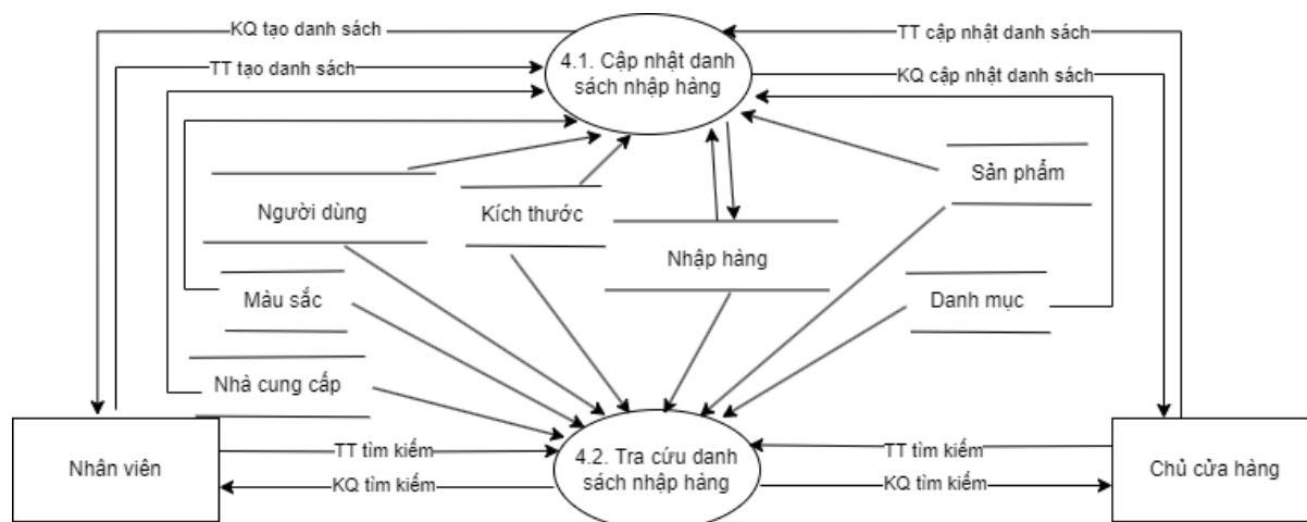
Hình 3.14. Sơ đồ luồng dữ liệu mức dưới đỉnh quản lý nhập hàng
