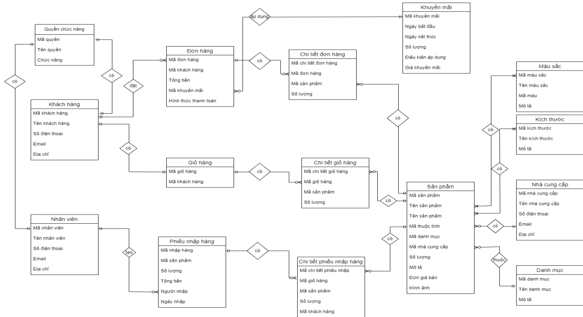
Hình 4.3. ERD hạn chế
