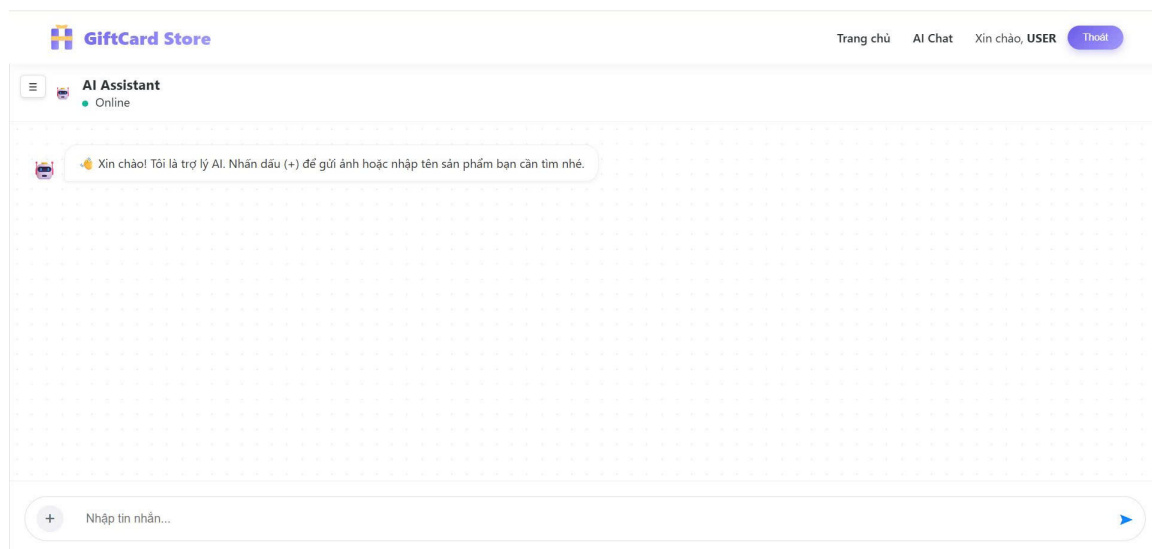
Hình 4.4: Trang Chatbot
