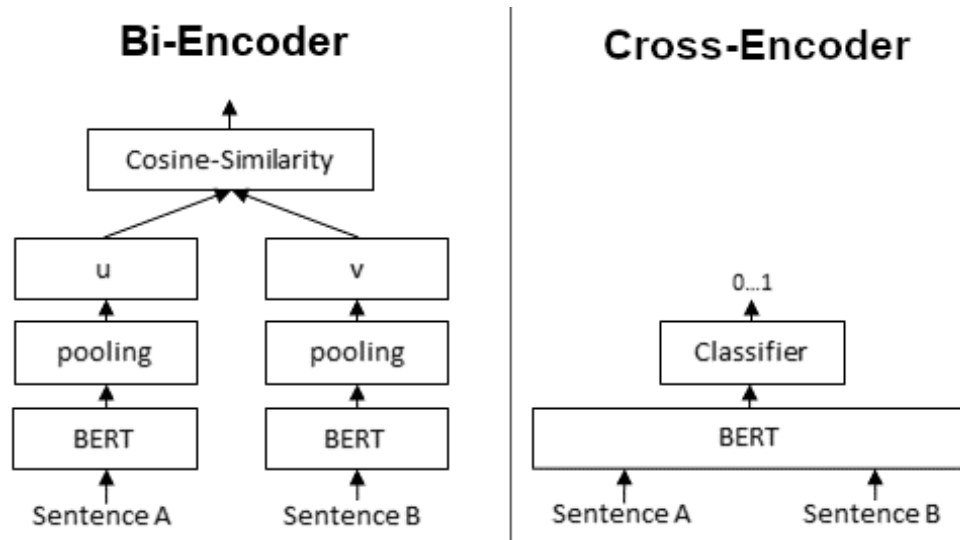
Hình 5.2: Sơ đồ so sánh kiến trúc giữa Bi-Encoder (trái) và Cross-Encoder (phải)
