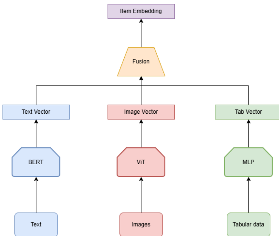
Hình 3.3: Kiến trúc Item Tower: Quy trình mã hóa và hợp nhất dữ liệu Đa phương thức
