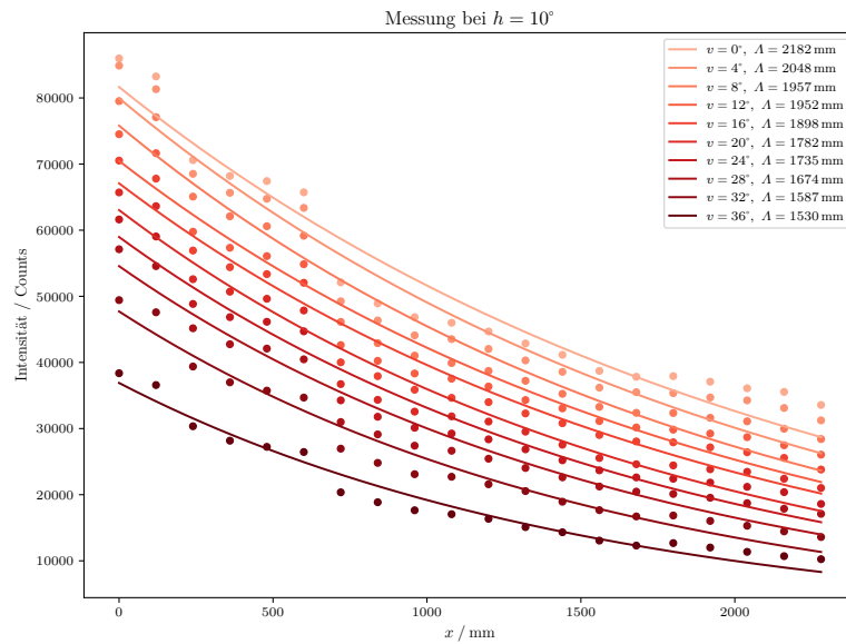
Abbildung 12: Die gemessenen Intensitäten für einen festen horizontalen Winkel h = 10^\circ und verschiedenen vertikalen Winkeln v von 0^\circ bis 36^\circ und verschiedenen x -Werten von 0 mm bis 2400 mm.
