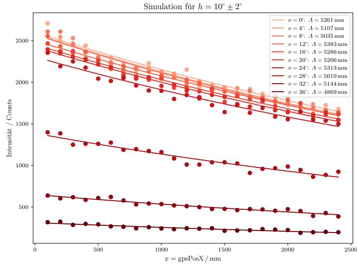
Abbildung 11: Die simulierte Intensität für einen festen horizontalen Winkelbereich h = 10^\circ \pm 2^\circ und verschiedenen vertikalen Winkelbereiche v von 0^\circ \pm 2^\circ bis 36^\circ \pm 2^\circ und verschiedenen "gpsPosX" Werten von 100 mm bis 2400 mm.
