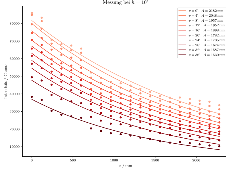
Abbildung 12: Die gemessenen Intensitäten für einen festen horizontalen Winkel h = 10^\circ und verschiedenen vertikalen Winkeln v von 0^\circ bis 36^\circ und verschiedenen x -Werten von 0 mm bis 2400 mm.
