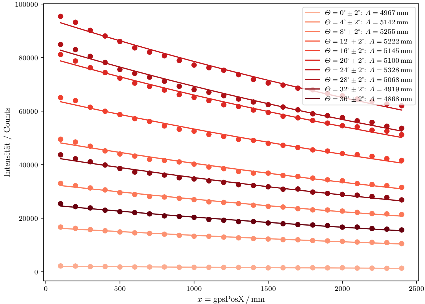
Simulation für verschiedene Winkel \Theta zur Faserachse
