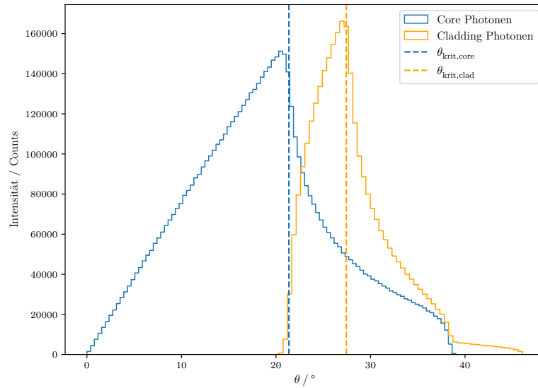
Abbildung 9: Die simulierten Intensitäten in ein Histogramm gegen den Winkel \Theta aufgetragen.
