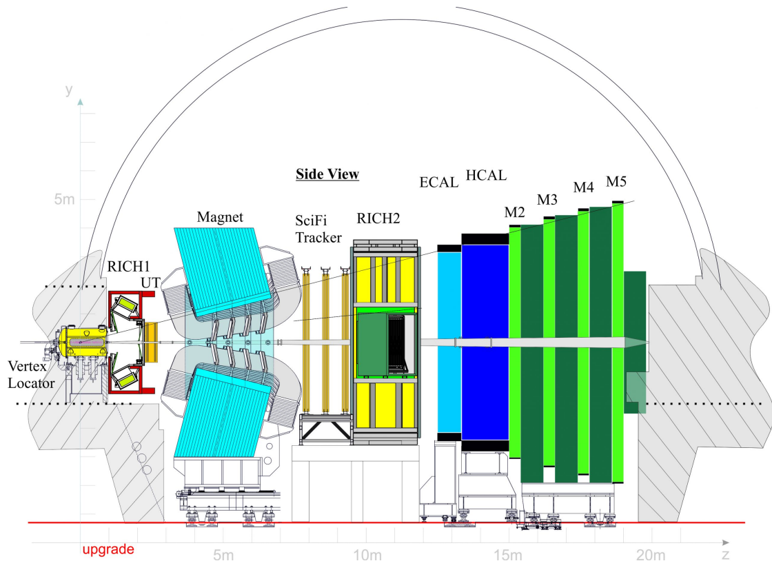
Abbildung 1: Schematische Darstellung eines Querschnittes des LHCb Upgrade 1 Detektors [2].
