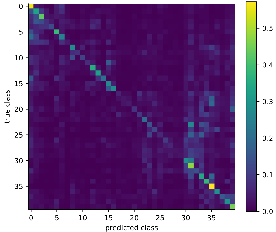
CORAL - NinaPro DB7
