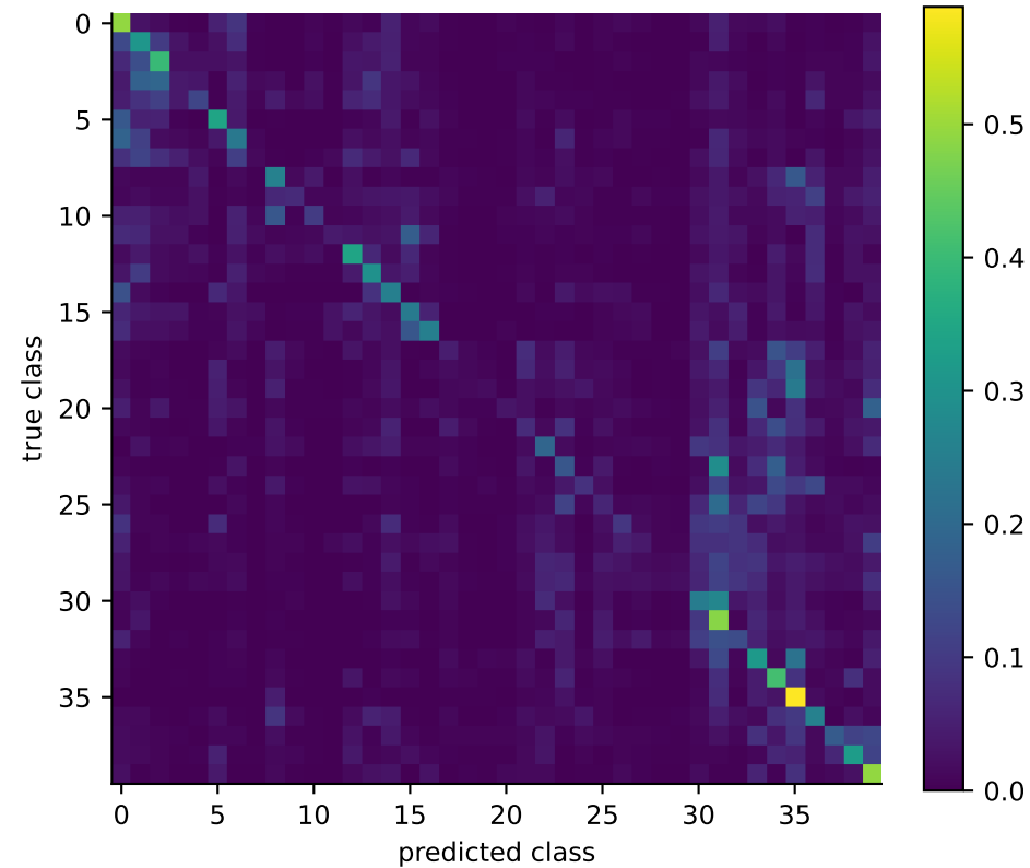
Raw - NinaPro DB7
