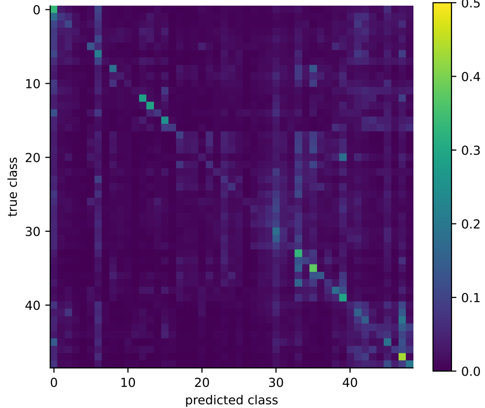
CORAL - NinaPro DB2
