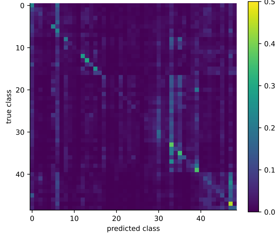
Raw - NinaPro DB2
