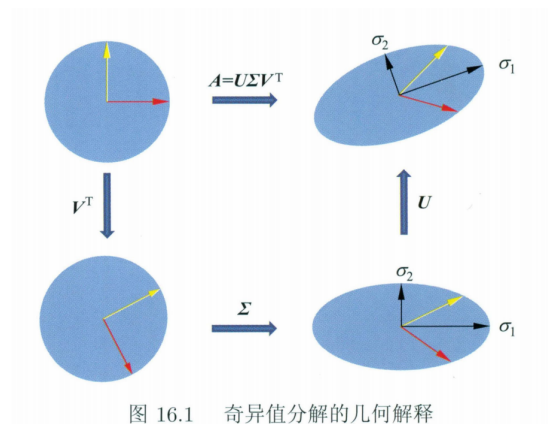
图 16.1 奇异值分解的几何解释
