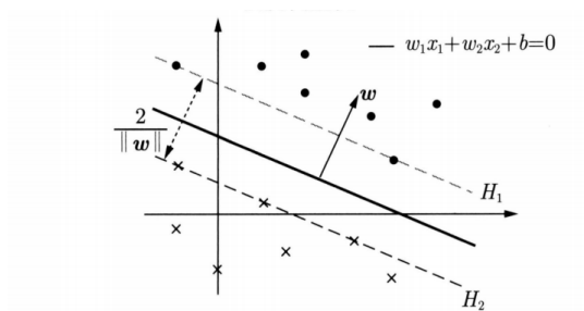
图 1: 支持向量示意图
