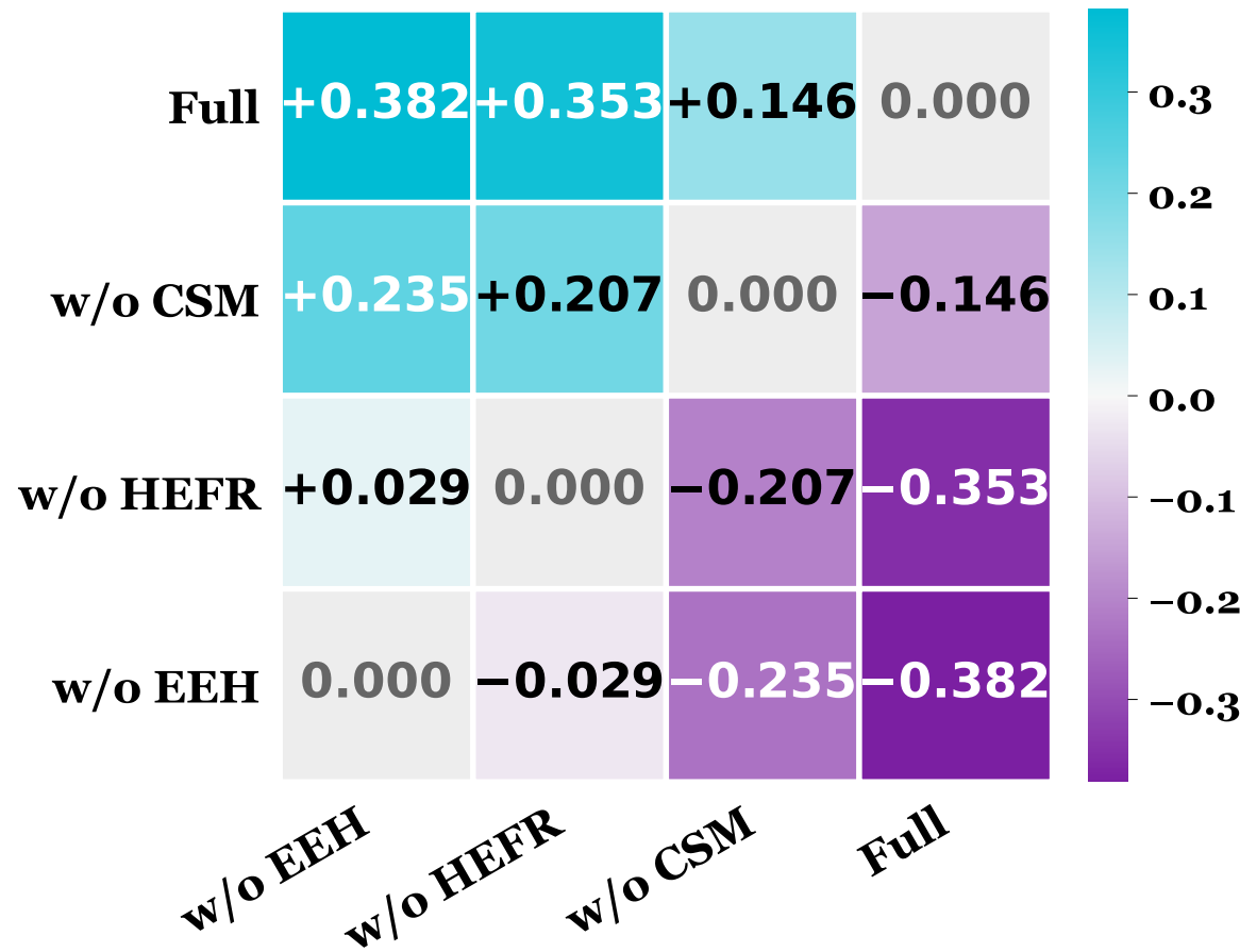
GPT-5.4-mini -- MCC
