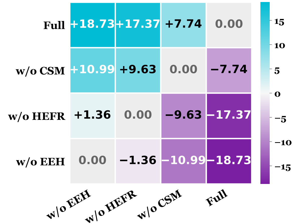
GPT-5.4-mini -- F1 (%)
