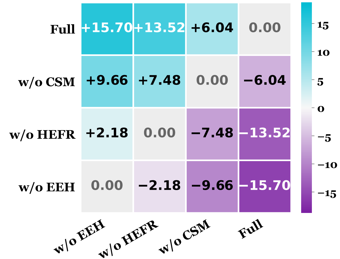
DeepSeek-V4-Flash -- F1 (%)
