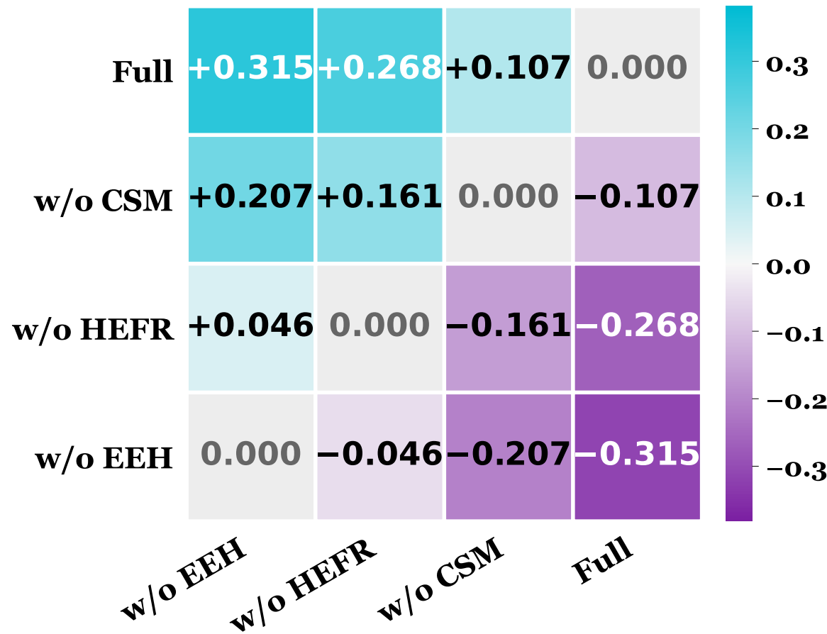
DeepSeek-V4-Flash -- MCC
