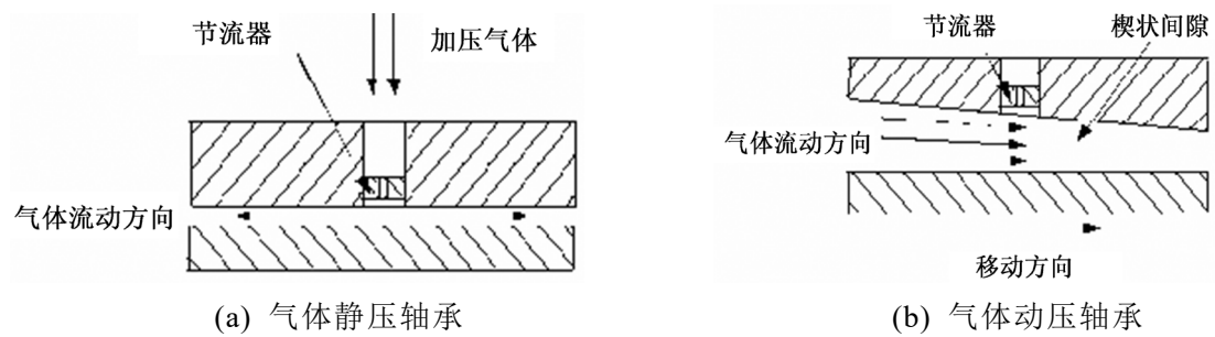
图 1-1 气体润滑轴承的分类
