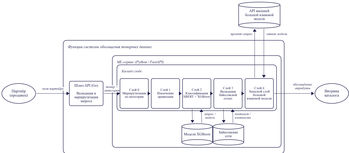
Рисунок 3 – Функциональная модель системы обогащения товарных данных
