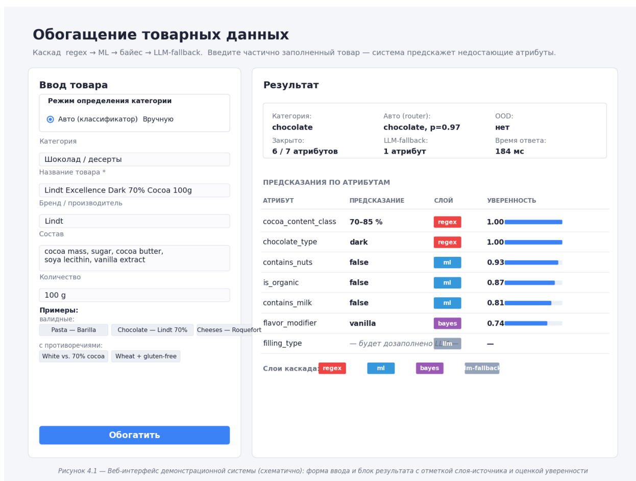
Рисунок 11 – Веб-интерфейс демонстрационной системы (схематично): форма ввода партнёр-доступных полей и блок результата с отметкой слоя-источника и оценкой уверенности на каждый атрибут
