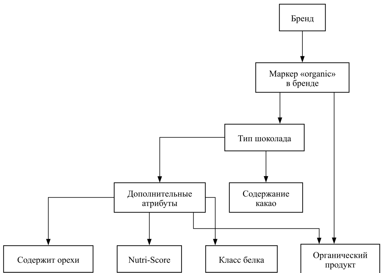
Рисунок 10 – Структура байесовской сети категории chocolate (направленный ациклический граф, обученный алгоритмом Hill Climb с критерием BIC)
