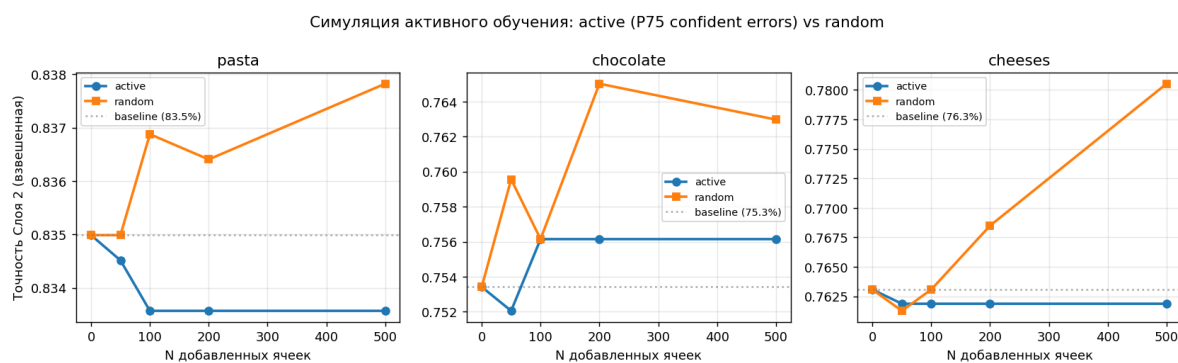
Рисунок 11 – Симуляция активного обучения: точность Слой 2 на holdout как функция количества добавленных gold-ячеек.
