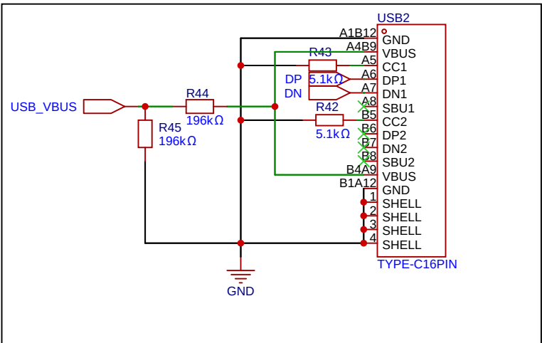
USB-C PWR
