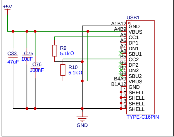
USB-C PWR
