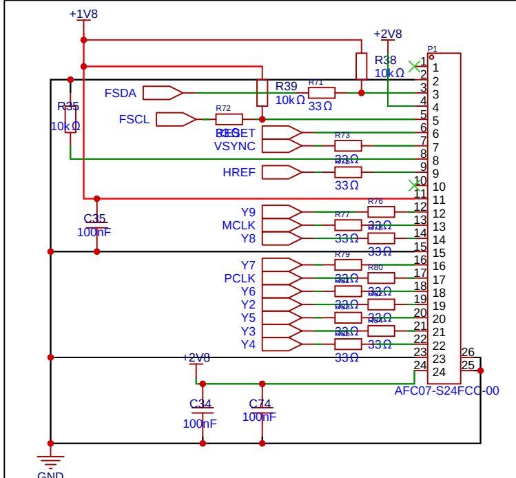
OV5640
