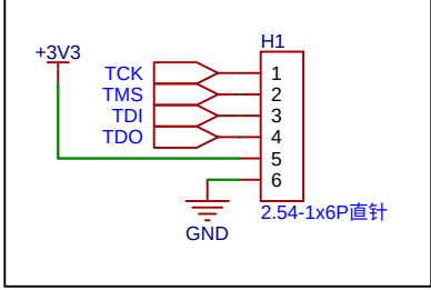
JTAG Header
