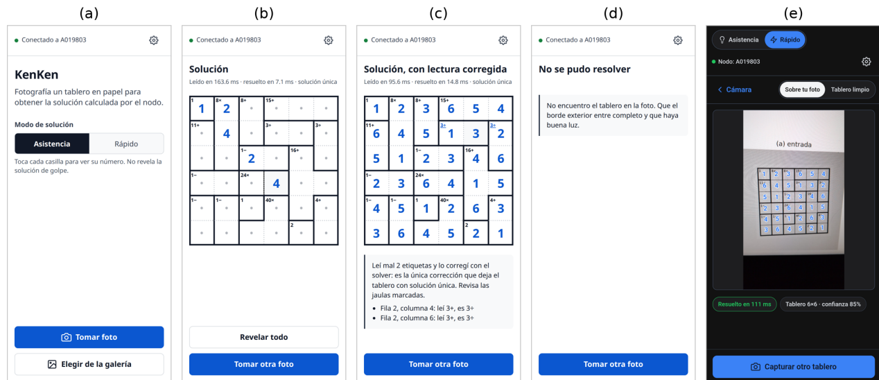
Figura 3. La app muestra lo que el solver decidió, incluida la corrección. (a) Inicio: estado del nodo y modo. (b) Modo Asistencia: el tablero sin números; la persona revela solo las casillas que toca. (c) Una foto de la Fig. 2a tomada a la pantalla: la visión leyó los dos 3÷ como 3+, el solver reparó la lectura y la app marca las jaulas corregidas. (d) Una foto cortada: el nodo no encuentra el tablero y lo dice en llano. (e) Captura del teléfono (Pixel 9a): en Modo Rápido, la solución aparece dibujada sobre la foto, cada número en su celda pese a la inclinación. Resolverla tomó 111 ms.
