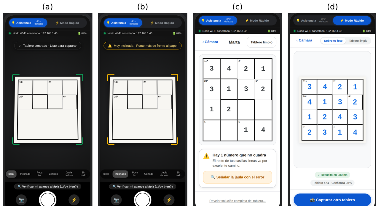
Figura 3. El prototipo de app lleva al verificador al usuario. (a) El visor confirma que el tablero está listo para capturar. (b) Avisa antes de capturar si la foto está inclinada. (c) Modo Asistencia, por defecto: verifica el avance a lápiz y señala que un número no cuadra, sin revelar la solución. (d) Modo Rápido: proyecta la solución sobre la foto. Capturas previas a la conexión con el nodo; tableros y tiempos son de ejemplo.
