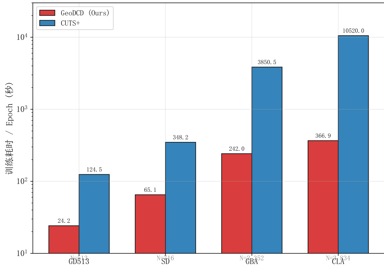
不同规模数据集上的训练效率对比
