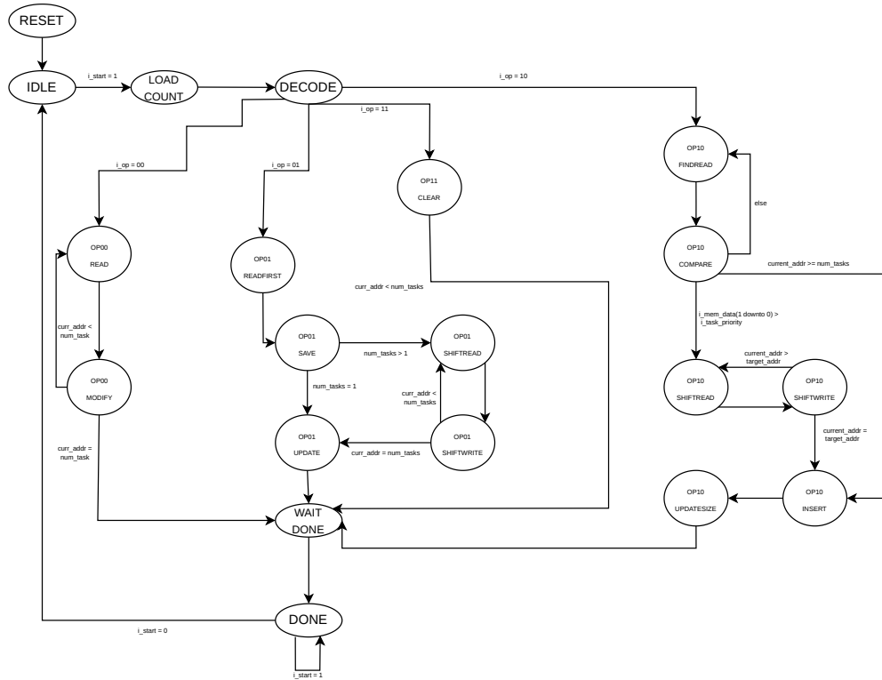
Figura 2: Schema dettagliato della FSM.
