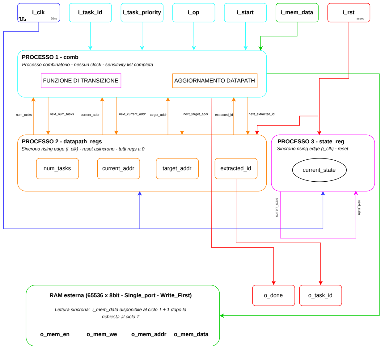
Figura 1: Schema a blocchi
