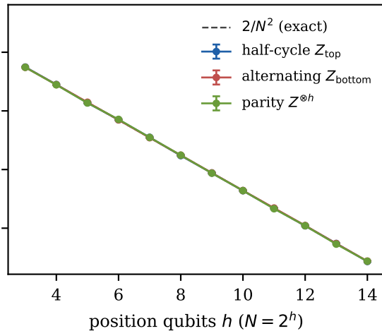
(b) Fourier-phase ansatz, N parameters
